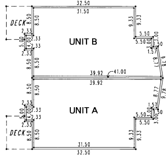
UPPER LEVEL SCALE: 1" = 20'
