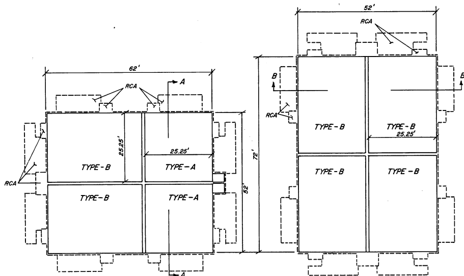
TYP. BLDG. PLANS, TYPE-AB BLDGS. 1, 2 & BLDGS. 5 THRU 12
